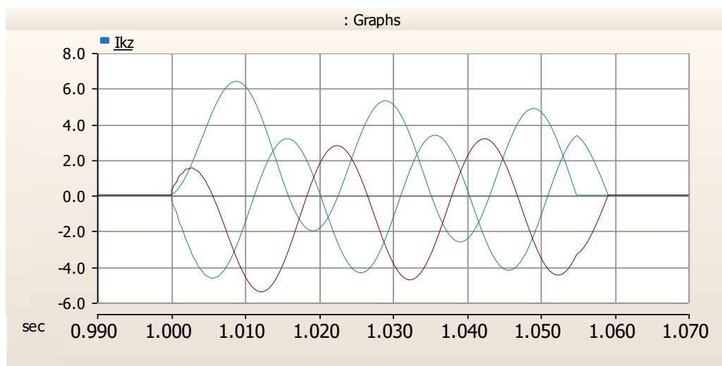
Рисунок 4. Осциллограмма трехфазного короткого замыкания в ПС PSCAD.
