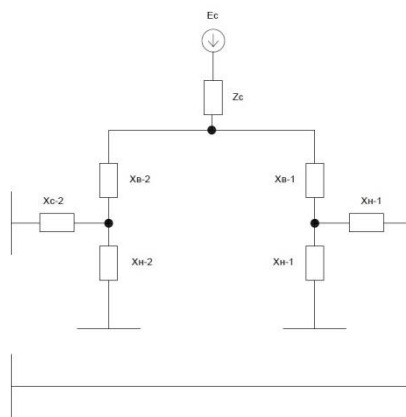
Рисунок 2. Схема замещения прямой последовательности для расчета ТКЗ в точках К1, К2 и К3.
