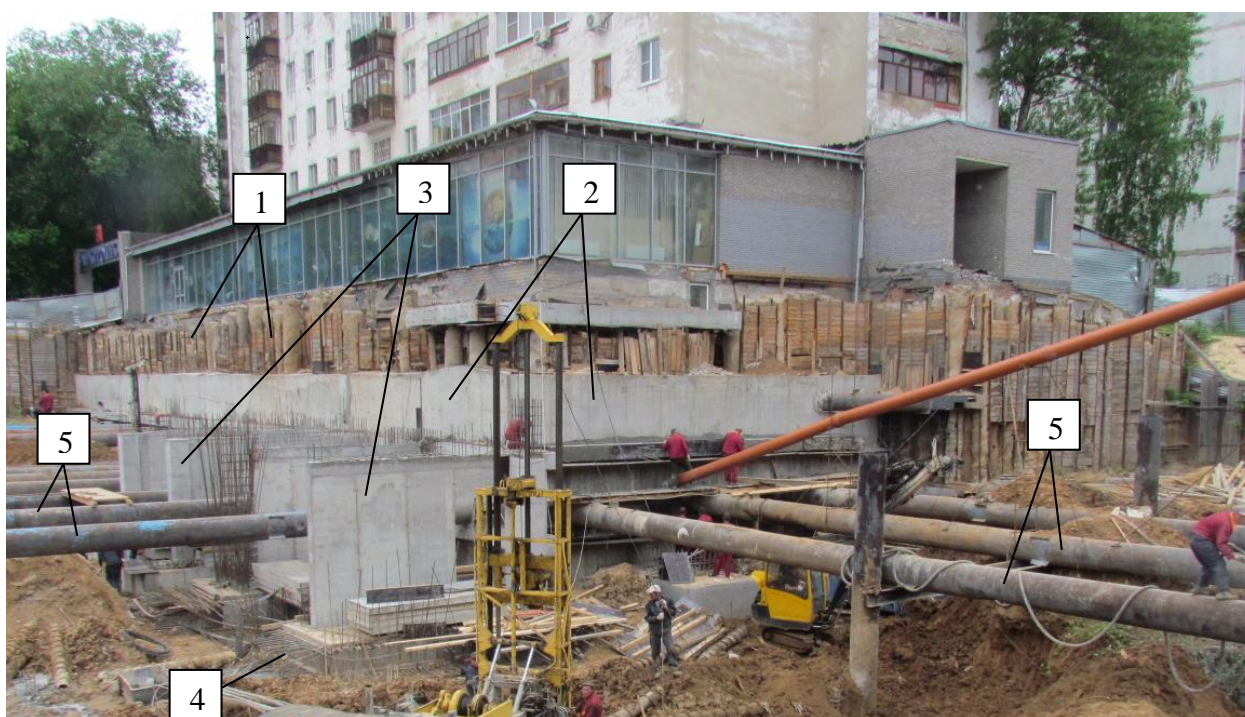
Рисунок 1. Схема закрепления подпорных стен котлована расстрелами из стальных труб 1000 мм: 1 - существующие буронабивные сваи ограждения котлована; 2 - ограждение котлована из монолитного железобетона; 3 - монолитные железобетонные контрфорсы усиления существующей подпорной стены; 4 - монолитный железобетонный ростверк; 5 - существующие трубы - расстрелы усиления подпорных стен
