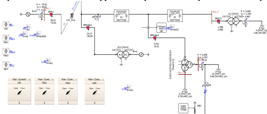
Рисунок 2. Исходная модель схемы в ПС PSCAD.
