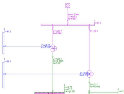
Рисунок 5. Короткое замыкание на шине низшего напряжения трансформатора Т2.
