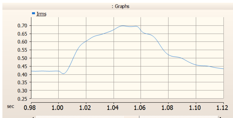
Рисунок 4. График изменения начального периодического действующего значения трехфазного ТКЗ в ПС PSCAD.
