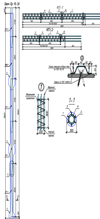
Рисунок 1. Пример схемы армирования буронабивной сваи-ЭРТ Ср-15-30 (15 – длина сваи в м., 30 – диаметр в см.). 1 - продольная арматура класса А500с; 2 – поперечная арматура класса А240; 3 – фиксатор каркаса сваи (из стальной пластины b=20 мм, t=4 мм; 4 - труба d159 мм обеспечивает жесткость каркаса при транспортировке и складировании; 5 – уширения вдоль ствола и пяты сваи.
