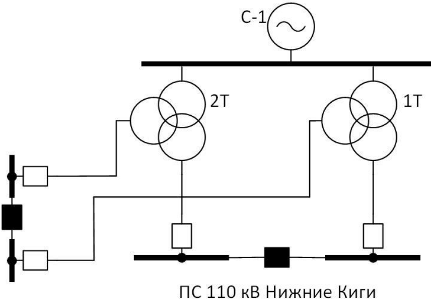
Рисунок 1. Исходная схема подстанции «Нижние Киги».
