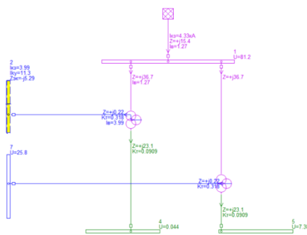
Рисунок 4. Короткое замыкание на шине среднего напряжения трансформатора Т2.
