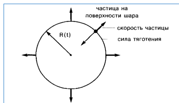
Рисунок 1. Расширяющийся однородный шар [17, с. 208]
