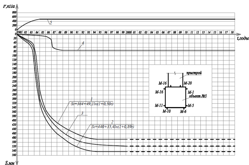
Рисунок 8. Объект №5. Графики изменения осадок фундамента во времени: 1 – минимальной; 2 – максимальной; 3 – средней; 4 – крена; 5 – средней осадки PIII
