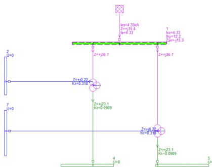
Рисунок 3. Короткое замыкание на шине системы.
