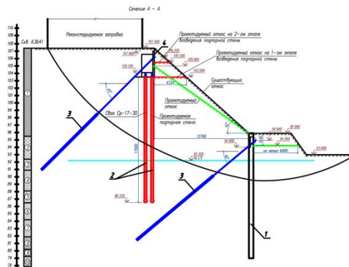
Рис. 2 Поперечное сечение прислоненного откоса с противооползневыми заглублен-ными железобетонными конструкциями: 1 - существующая подпорная стена из буронабивных свай диаметром 500,0 мм; 2 - буроинъекционные сваи ЭРТ усиления основания в два ряда; 3 - грунтовые анкера ЭРТ усиления склона; 4 - монолитная уголкоя же-лезобетонная подпорная стена.
