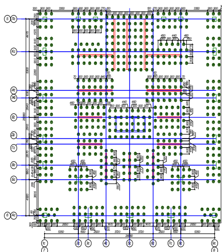
Рисунок 2 Свайное поле из погружаемых забивкой свай С 15.30-10.1
