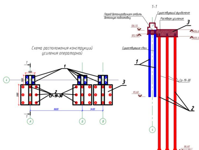
Рисунок 4 Схема усиления основания фундаментов операторной: 1 - существующие забивные сваи; 2 - буронагрейционные сваи ЭРТ; 3 - подводящая монолитная железобетонные консольные балки под существующие железобетонные ростверки.
