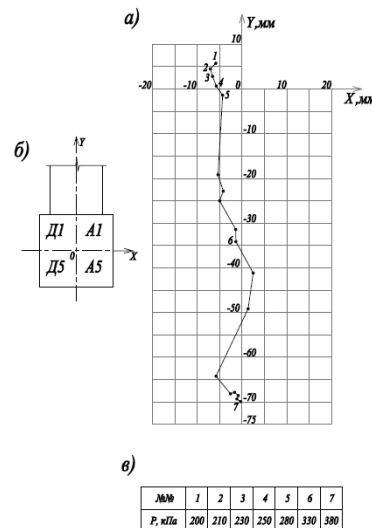
Рисунок 11. Объект №5. а - график изменения величины и направления неравномерной осадки; б – схема разбивки фундамента на квадраты; в – таблица роста среднего давления на основание
