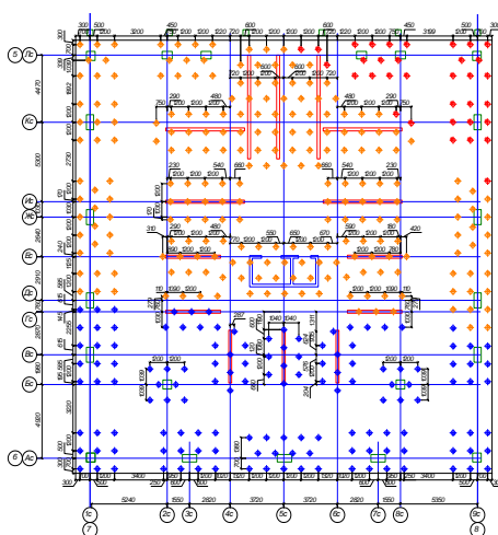
Рисунок 3 Свайное поле из буроньекционных свай ЭРТ
