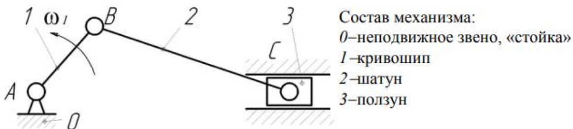
Рисунок 1. Кинематическая схема четырехзвенного кривошипно-ползунного механизма.
