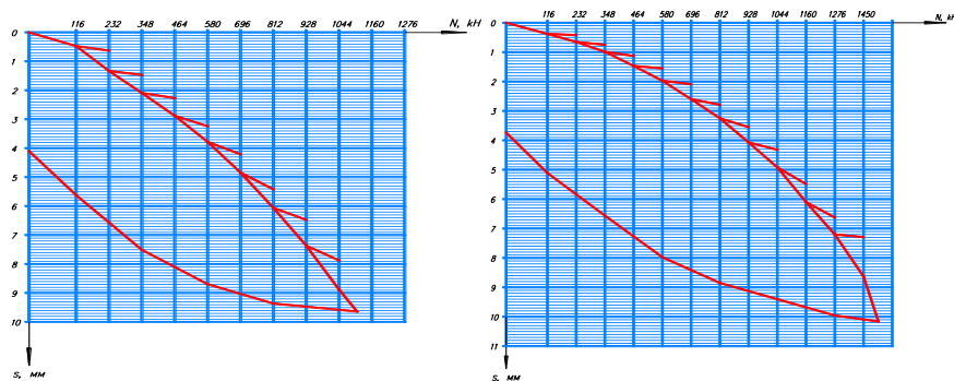
Рисунок 4 Графики зависимости осадки сваи ЭРТ S от нагрузки N : а – свая №101; б – свая №25.
