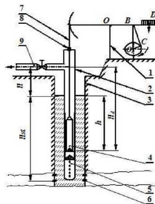
Рисунок 1. Принципиальная схема штанговой глубинно-насосной установки.
