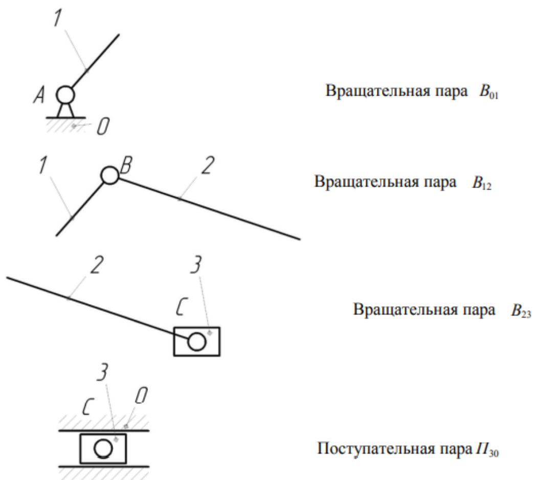
Рисунок 2. Кинематические пары
