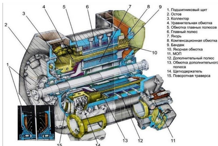
Рисунок 1 – Тяговый электродвигатель коллекторного типа и его устройство
