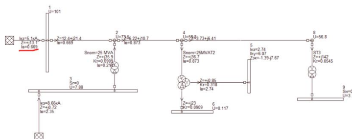
Рисунок 6. Проверка сходимости расчетов в ПК EnergyCS ТКЗ.
