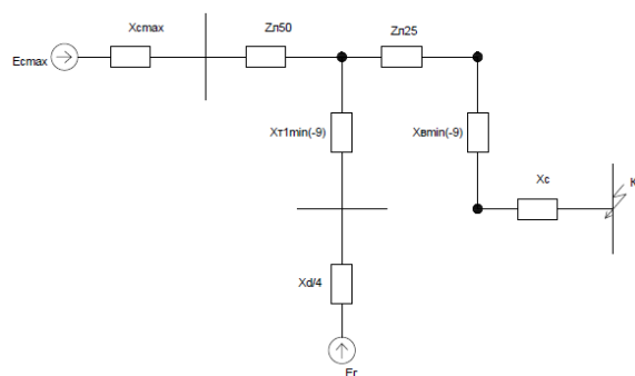
Рисунок 5. Схема замещения ПП для РТКЗ.
