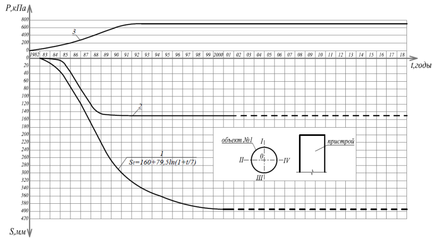
Рисунок 1 Объект №1. Графики: 1 – средней осадки; 2 –крена; 3 – роста среднего давления на основание.
