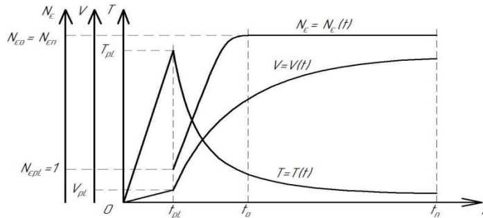
Рисунок 2. Возможный ход кривых V = V(t) , T = T(t) и \mathcal{N}_{\epsilon} = \mathcal{N}_{\epsilon}(t)
