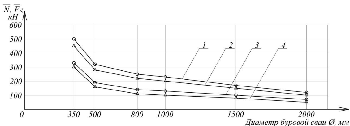
Рисунок 4 Графики зависимости f(\varnothing, \bar{N}) и f(\varnothing, \bar{F}_d) .
