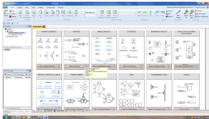
Рисунок 3. Библиотека компонентов ПС PSCAD.
