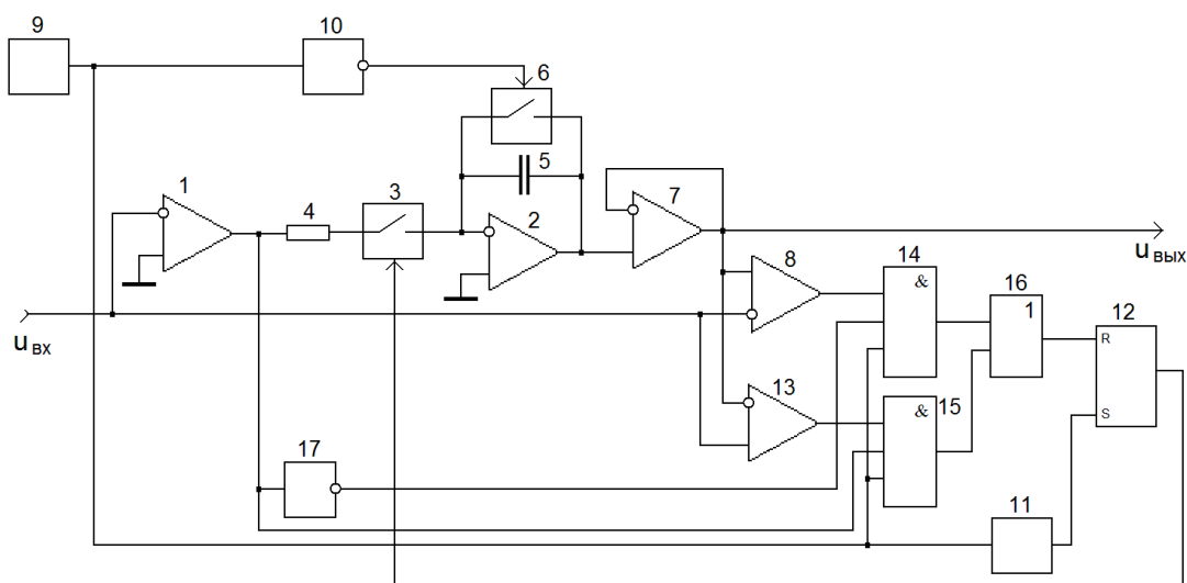
Рисунок 1. Схема устройства
