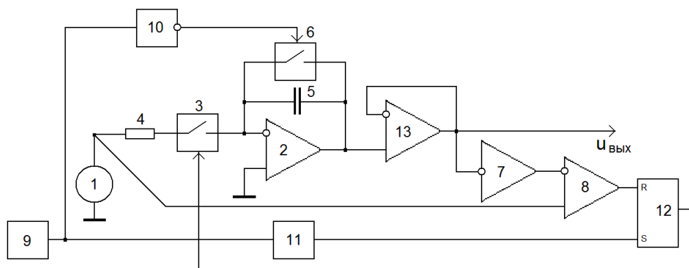
Рисунок 1. Схема устройства
